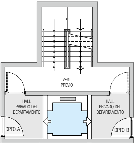
Ascensor con Doble embarque a 180°
