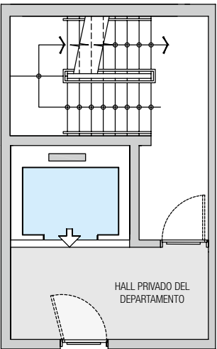
Ascensor con Simple embarque a 0°
